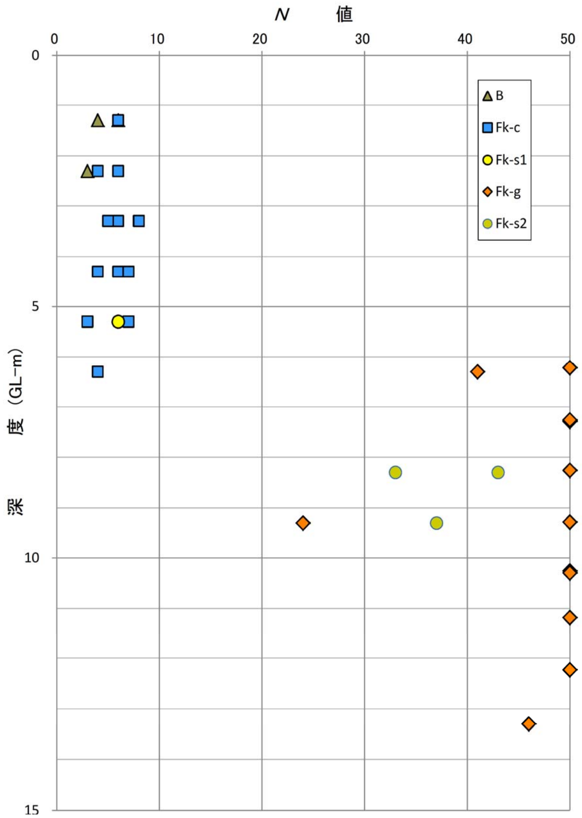
図 4.3 N値の深度分布
