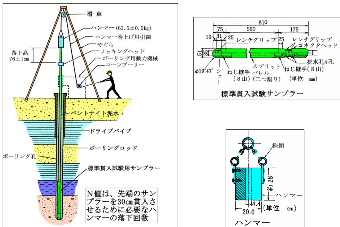
図 2.3 標準貫入試験装置概要図
